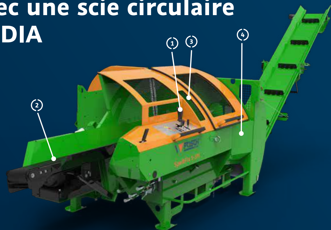
SpaltFix S-375
